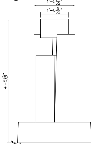
2 ELEVATION
